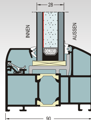
ISOGLAS U_g = 1,1 \text{ W/m}^2\text{K} Seitenteilverglasung - STANDARD
